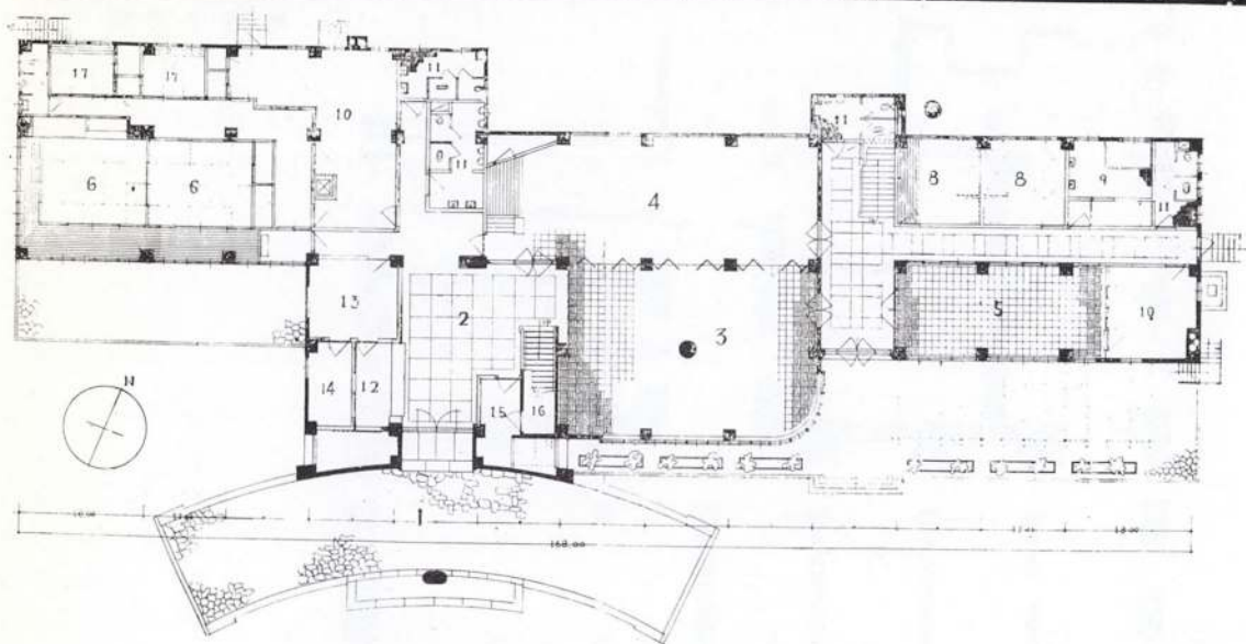
一階平面圖
