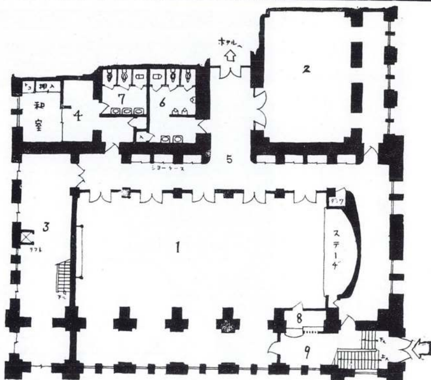
一階平面圖
