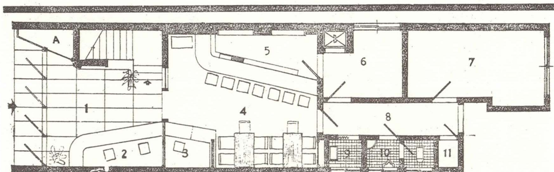
一階平面図
