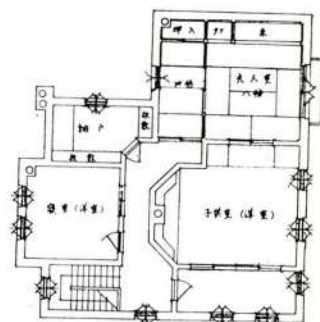
第2階平面圖 (112.125 m 2 )
