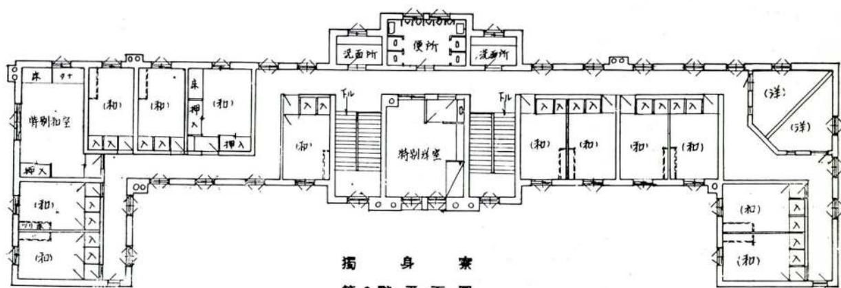
第2階平面圖
