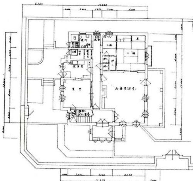
第1階平面圖 (135.500 m 2 )
